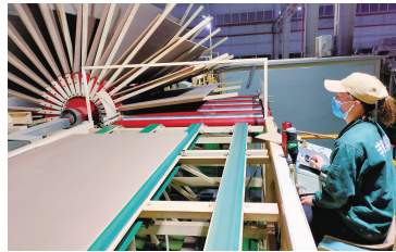
自动检板系统
